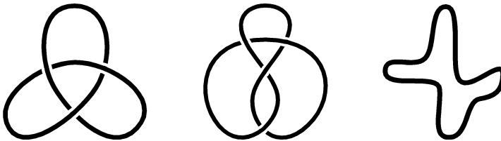
Рис. 1.1. Трилистник, восьмерка и тривиальный узел
